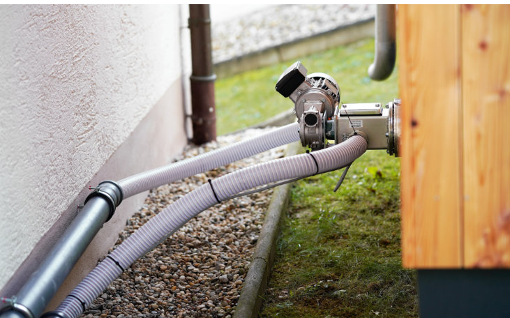
Verschiedene Anschlussmöglichkeiten zum Heizraum
